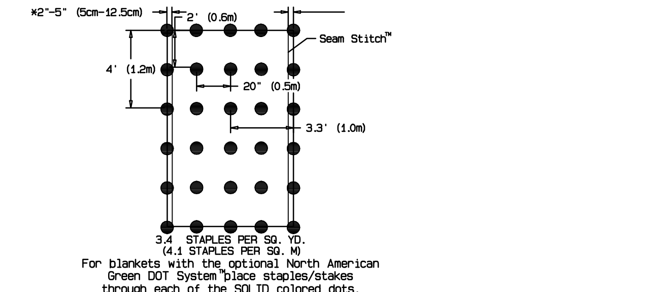
STAPLE PATTERN (D) DETAIL (USE WITH NAG S-75 LINING)
